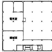
塔屋1階平面
