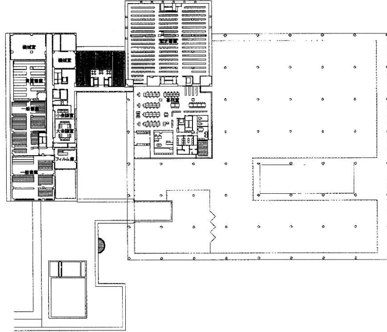
2階平面
