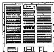
4階・中3階平面
